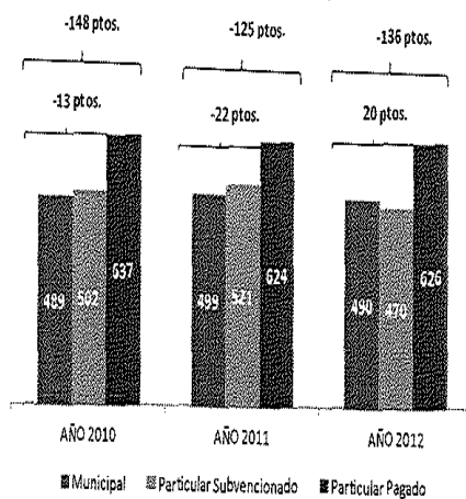
Evolución promedios PSU según dependencia
