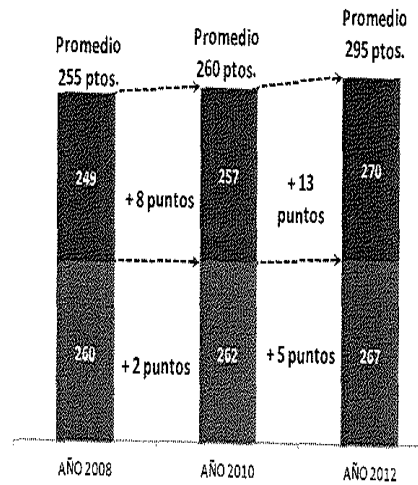
Evolución SIMCE 2° Medio últimos 4 años
