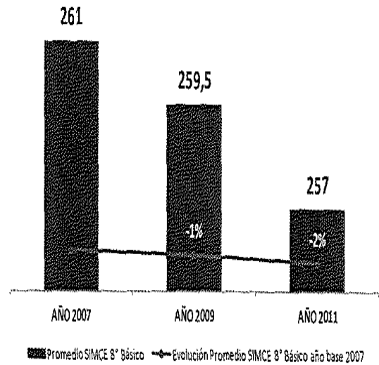
Evolución promedios SIMCE 8° Básico
