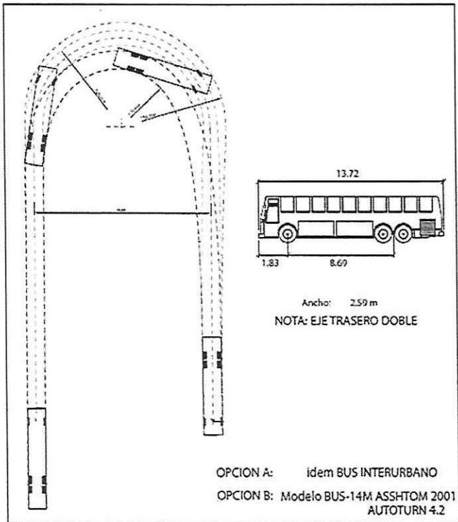
Imagen 2: Radios de Giros mínimos y máximos Bus Interurbano de eje trasero doble, REDEVU 2009.
